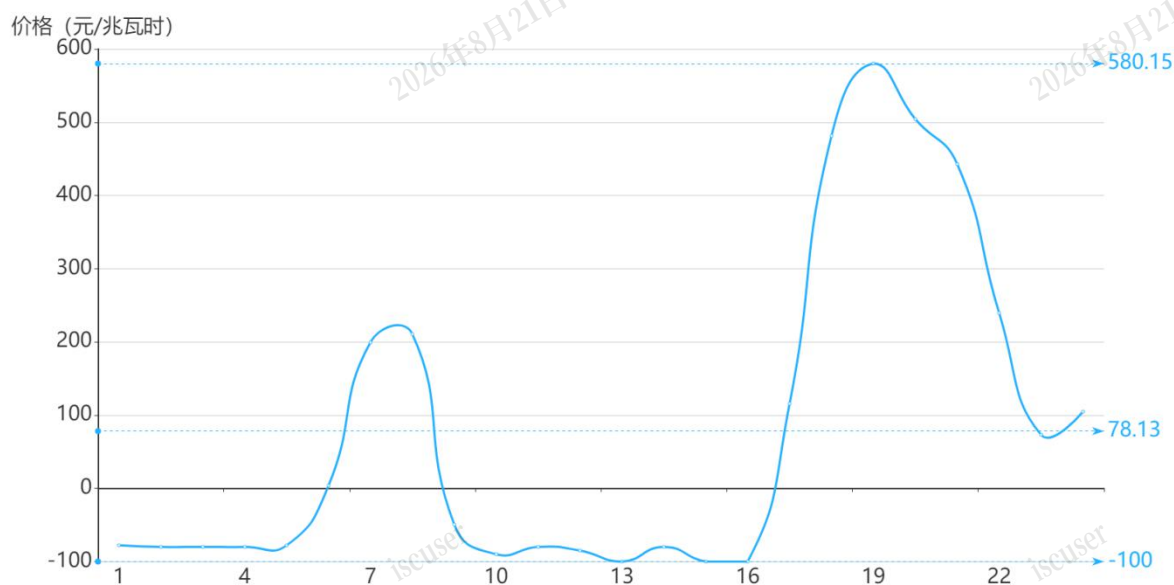
图3 3月19日实时市场用电侧价格
