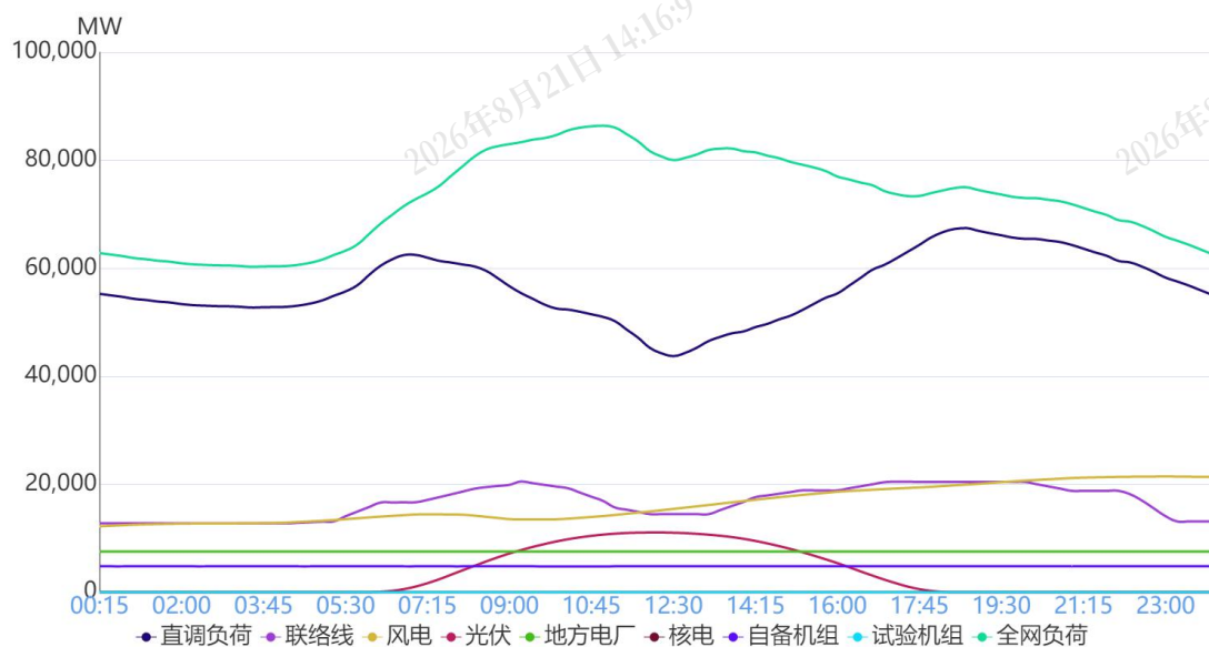
图 1 3月21日负荷及电源出力预测情况
