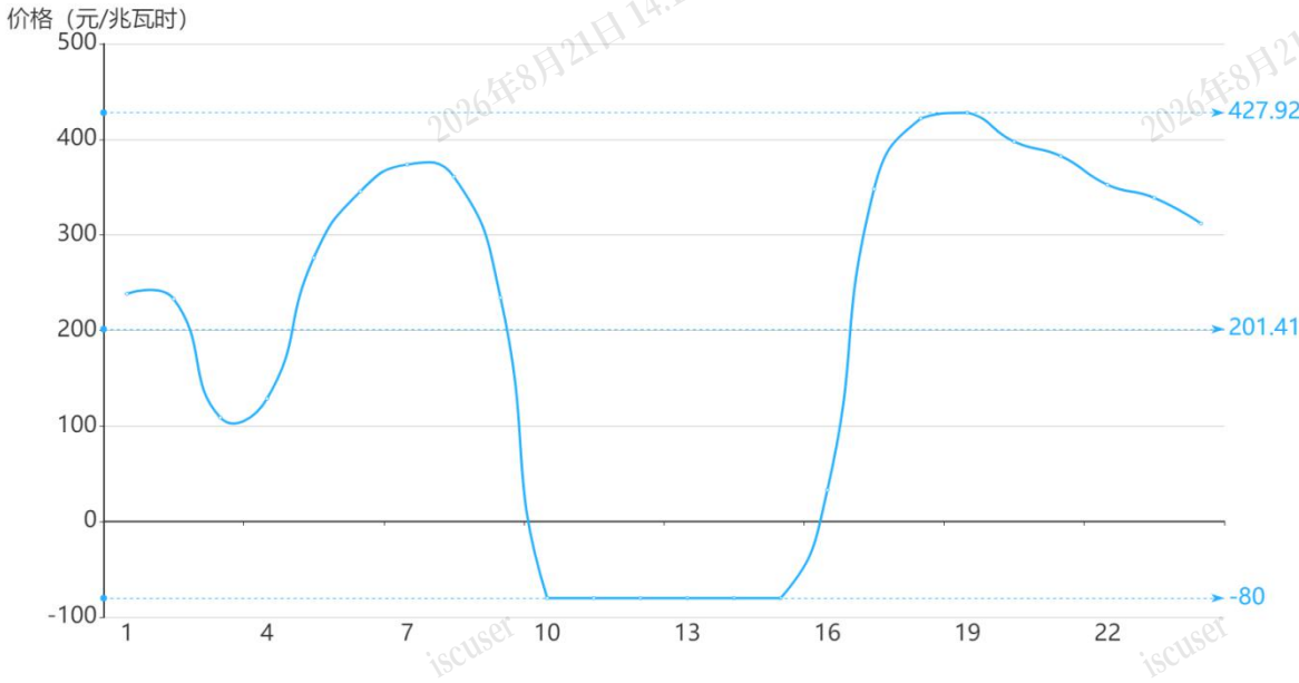
图 2 3 月 29 日日前市场用电侧价格
