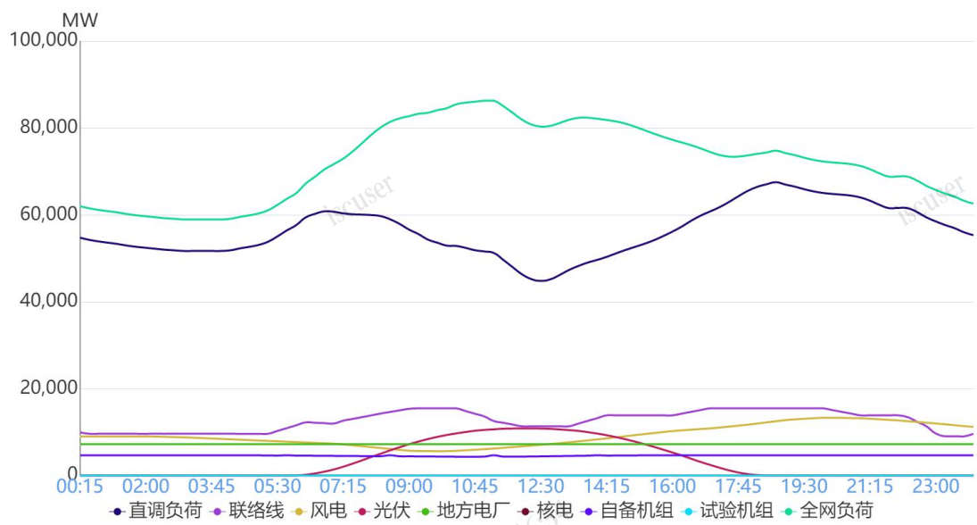
图 1 4 月 1 日负荷及电源出力预测情况
