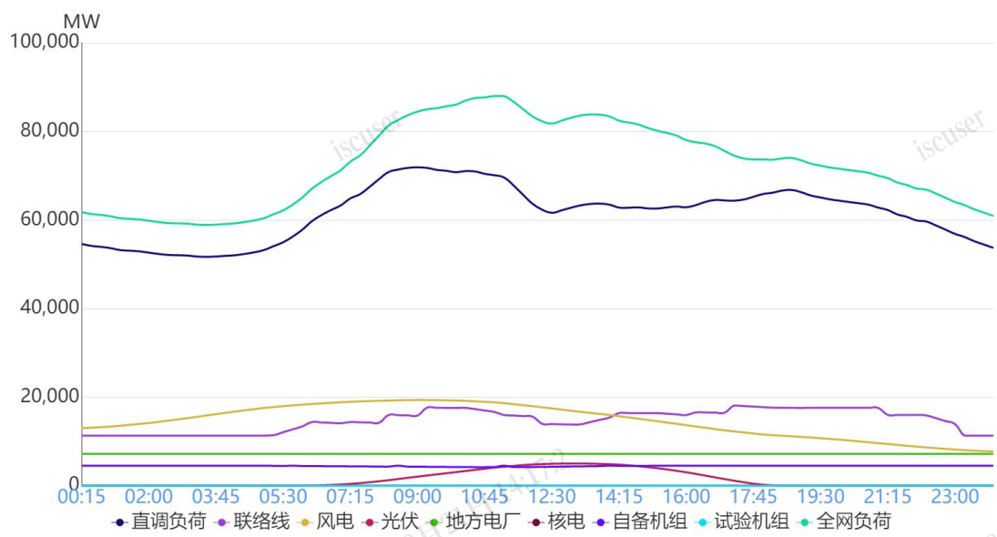
图 1 4月3日负荷及电源出力预测情况
