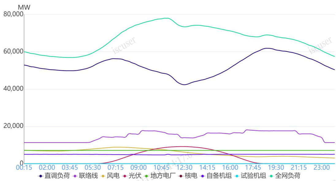
图 1 4月4日负荷及电源出力预测情况
