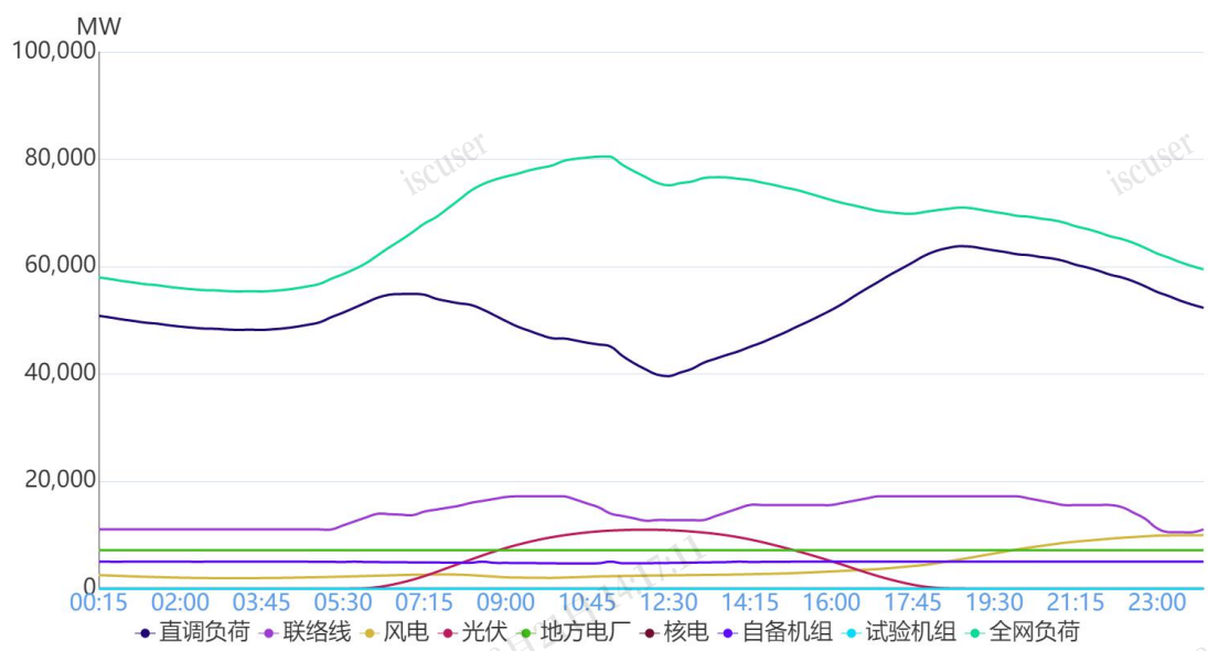
图 1 4月5日负荷及电源出力预测情况
