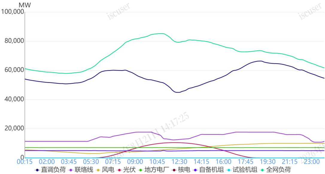
图 1 4月8日负荷及电源出力预测情况
