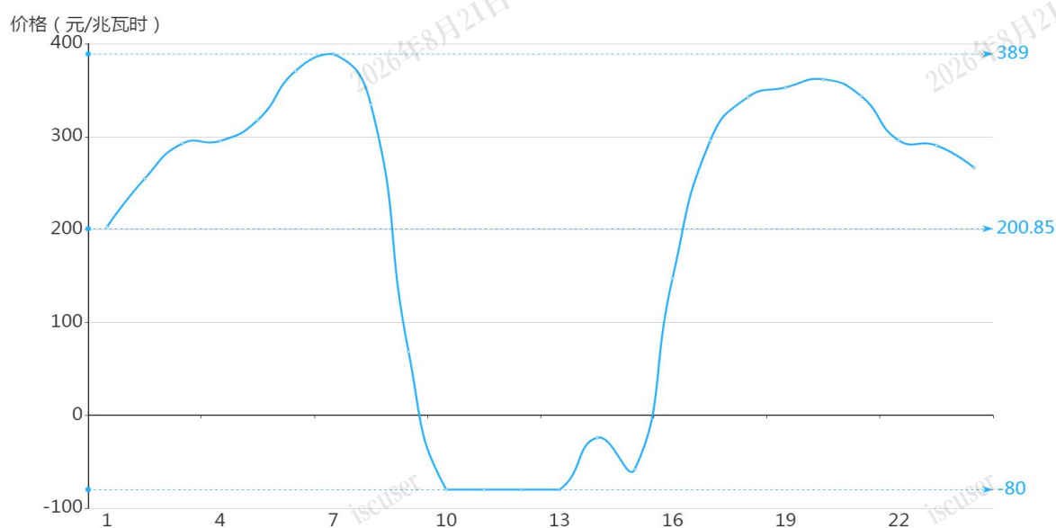
图3 4月12日实时市场用电侧价格
