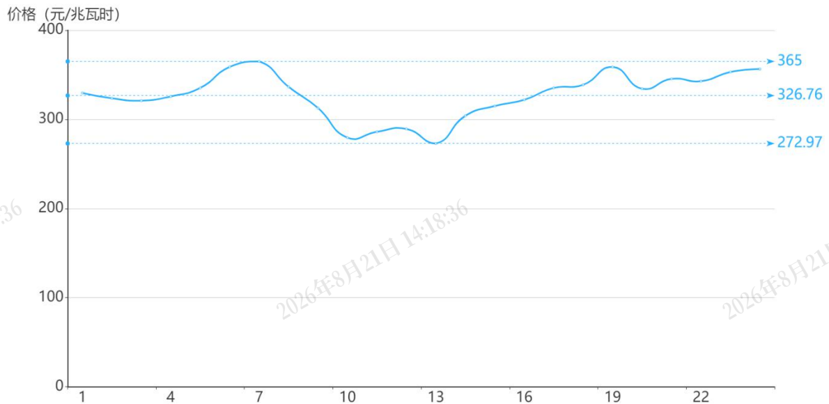
图2 4月19日日前市场用电侧价格
