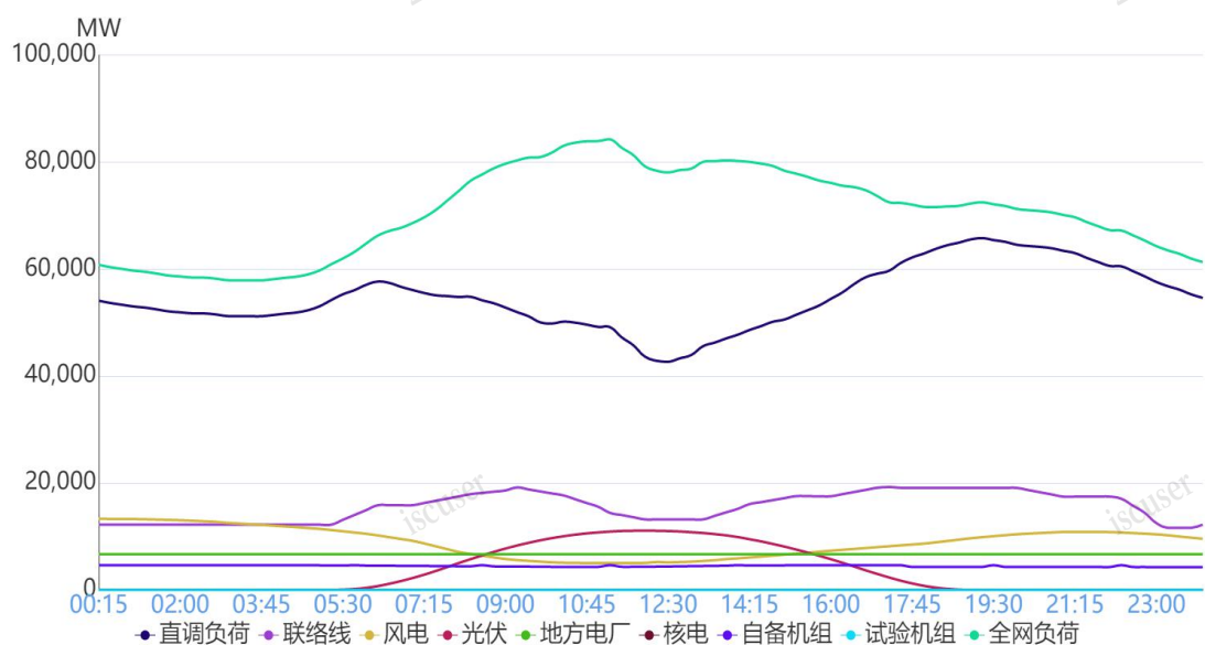
图 1 4月27日负荷及电源出力预测情况
