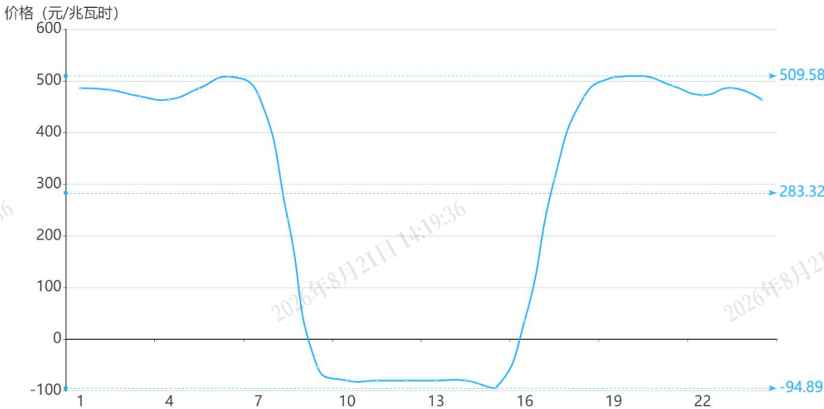
图3 5月1日实时市场用电侧价格
