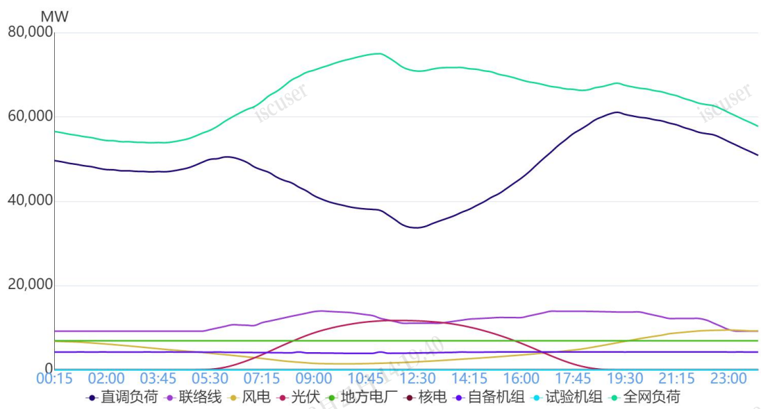
图 1 5月3日负荷及电源出力预测情况
