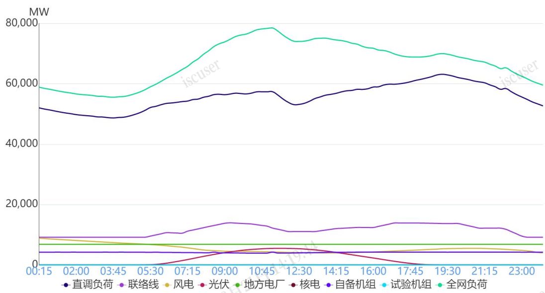
图 1 5月4日负荷及电源出力预测情况
