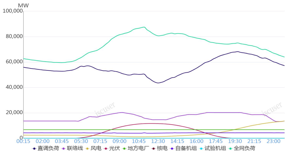
图 1 5月28日负荷及电源出力预测情况
