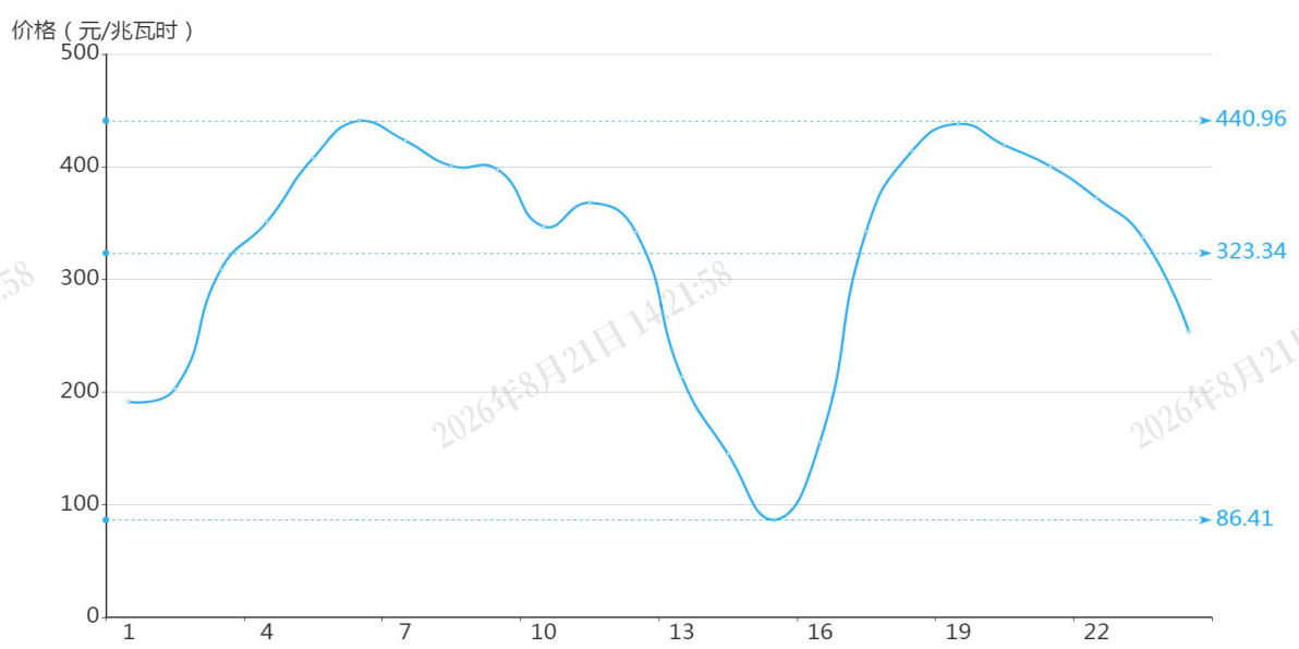
图3 5月30日实时市场用电侧价格
