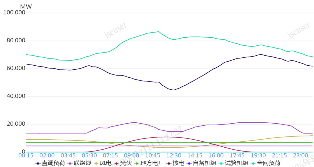
图 1 6月6日负荷及电源出力预测情况
