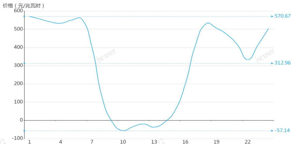
图2 6月6日日前市场用电侧价格
