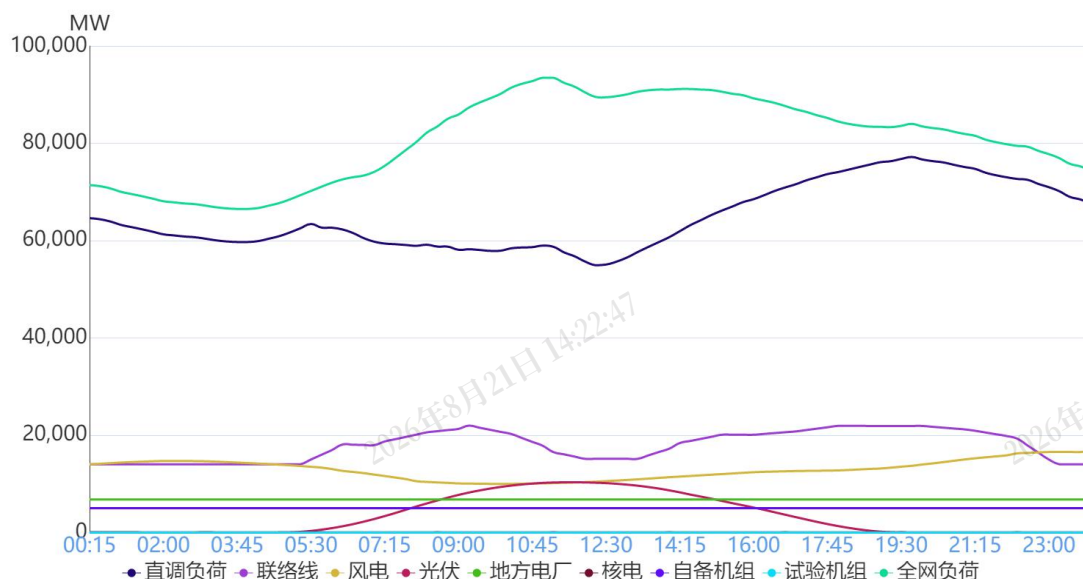
图 1 6月11日负荷及电源出力预测情况
