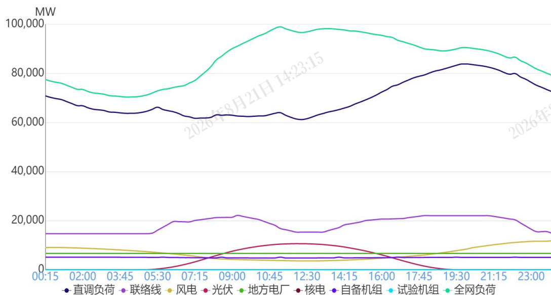
图1 6月17日负荷及电源出力预测情况
