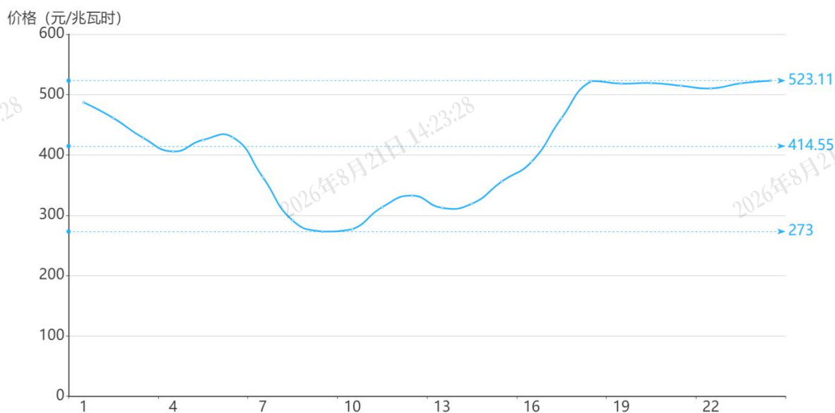
图 2 6月20日日前市场用电侧价格
