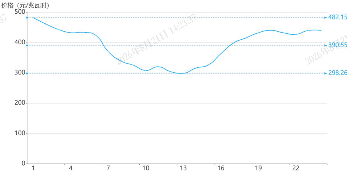
图 2 6 月 22 日日前市场用电侧价格
