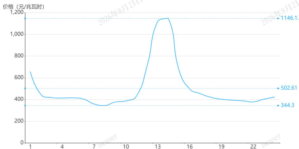
图3 6月21日实时市场用电侧价格
