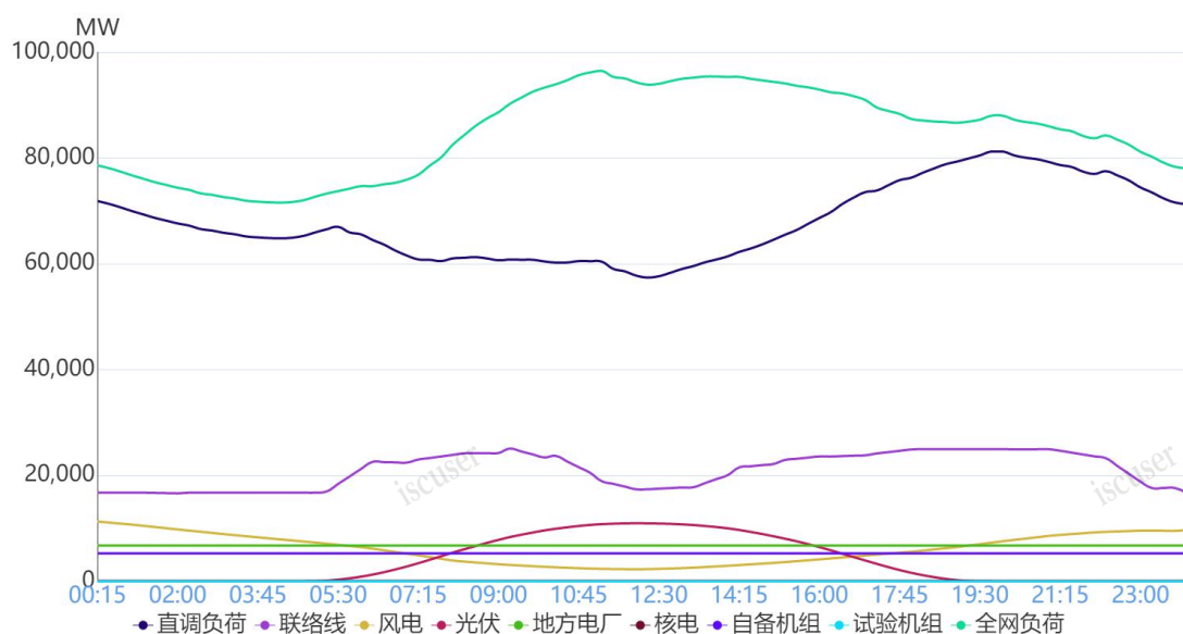
图1 6月27日负荷及电源出力预测情况
