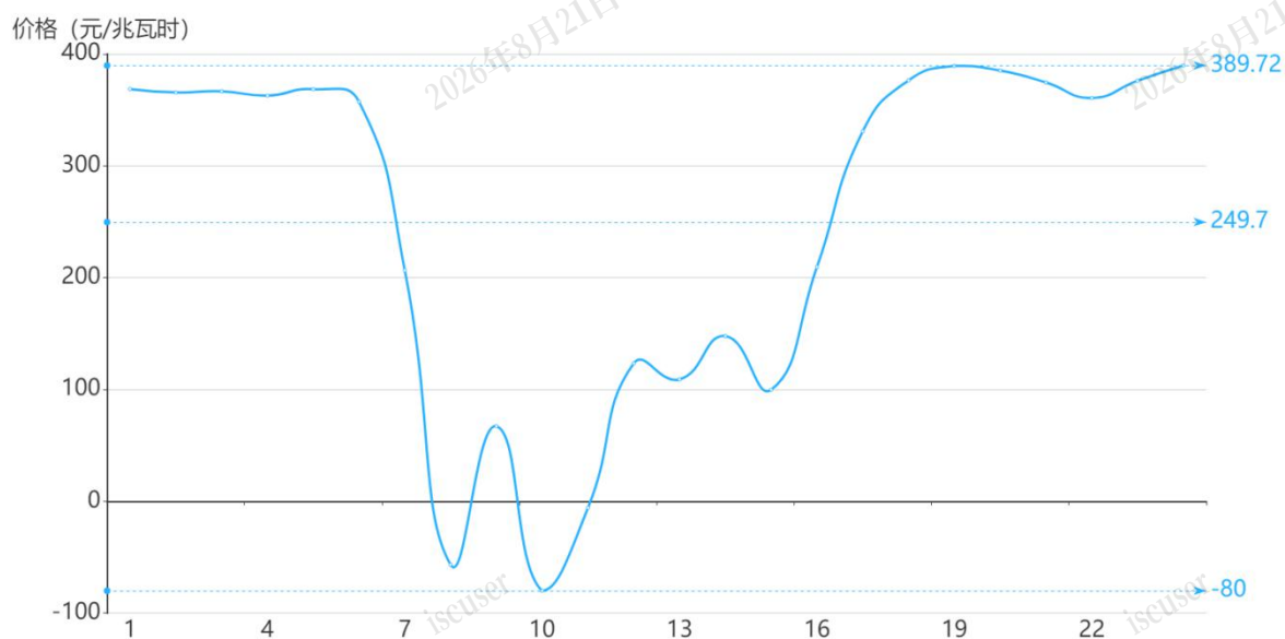
图3 6月27日实时市场用电侧价格
