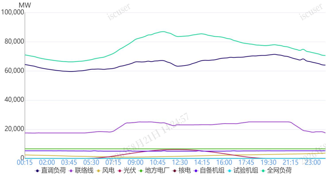
图 1 7月8日负荷及电源出力预测情况
