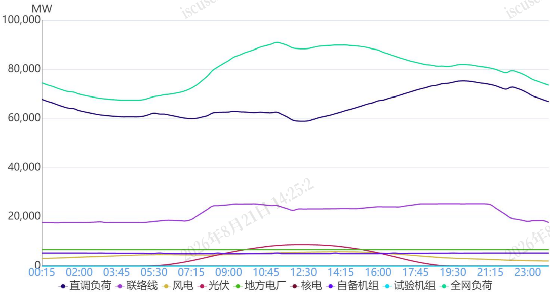
图 1 7月9日负荷及电源出力预测情况
