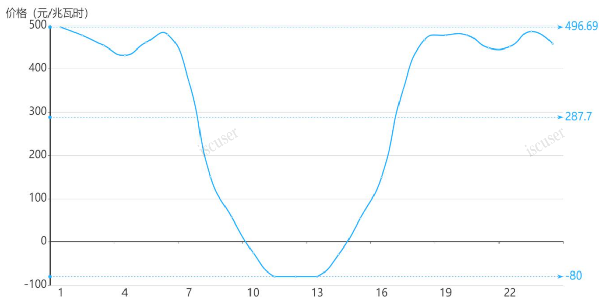
图2 7月12日日前市场用电侧价格
