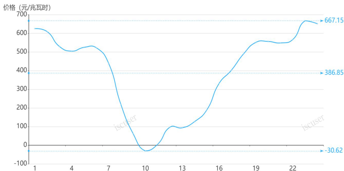
图 3 7 月 14 日实时市场用电侧价格
