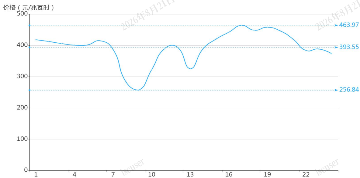
图3 7月19日实时市场用电侧价格
