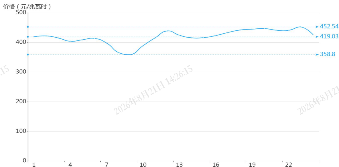
图 2 7 月 20 日日前市场用电侧价格
