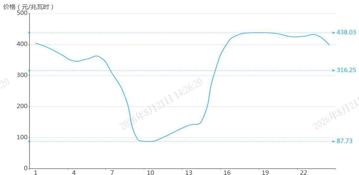
图 2 7 月 21 日日前市场用电侧价格
