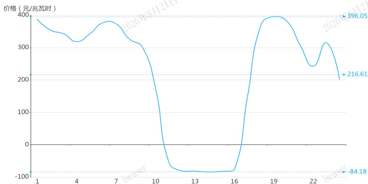
图 3 7 月 20 日实时市场用电侧价格
