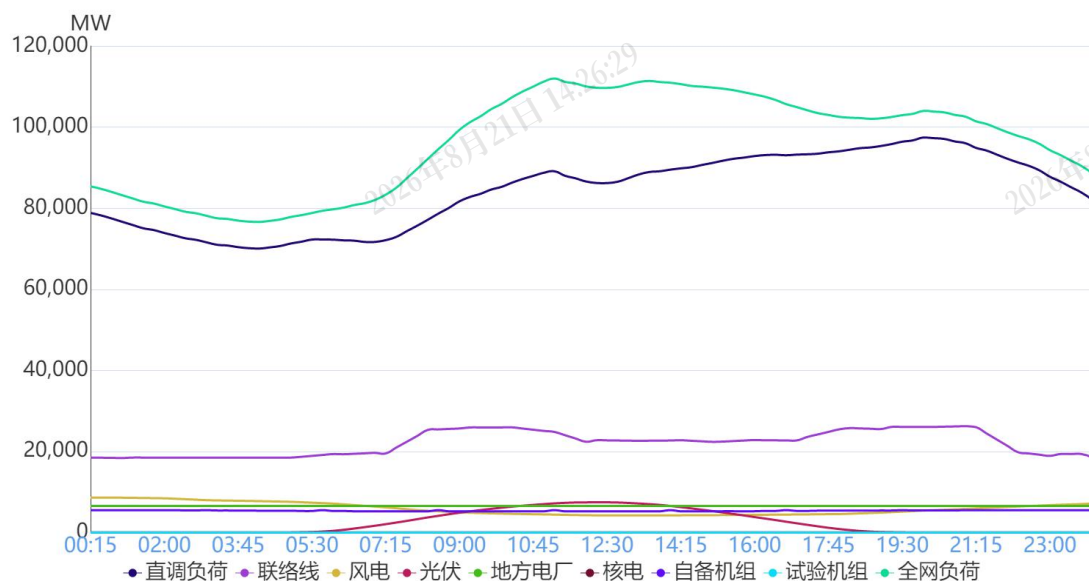
图 1 7月23日负荷及电源出力预测情况
