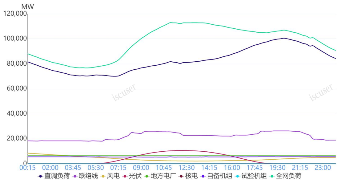
图 1 8 月 2 日负荷及电源出力预测情况
