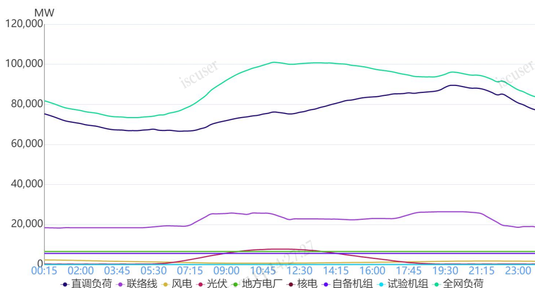
图 1 8月7日负荷及电源出力预测情况
