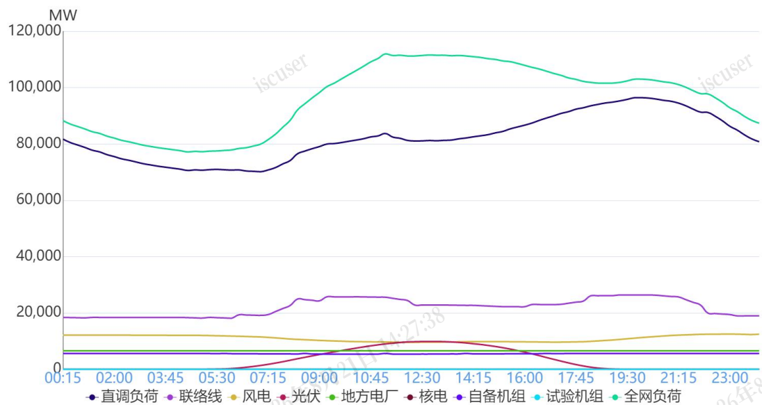
图 1 8月10日负荷及电源出力预测情况
