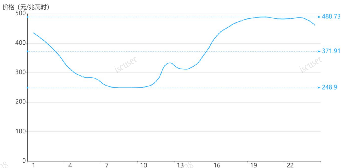
图2 8月10日日前市场用电侧价格
