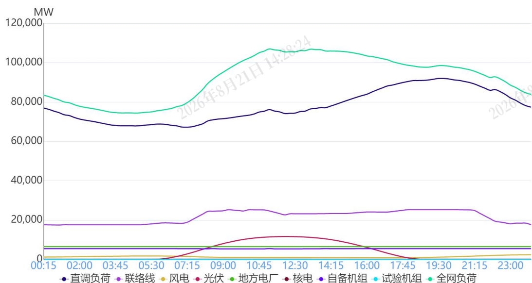
图 1 8月22日负荷及电源出力预测情况
