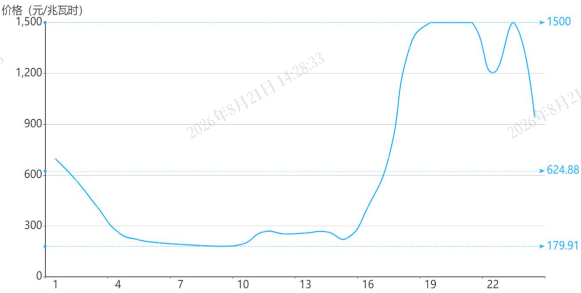
图 2 8 月 24 日日前市场用电侧价格
