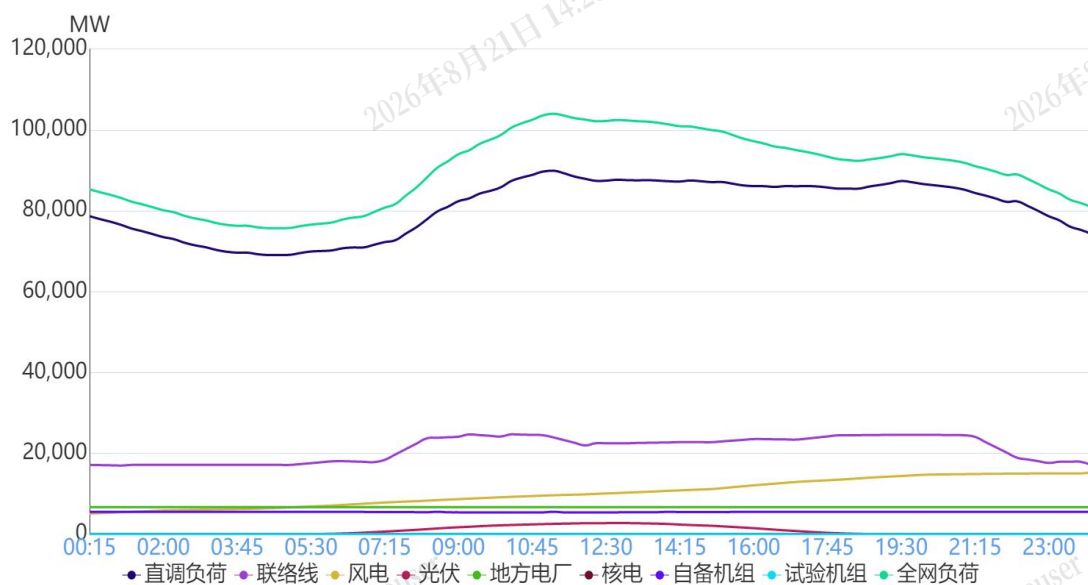
图 1 8月26日负荷及电源出力预测情况
