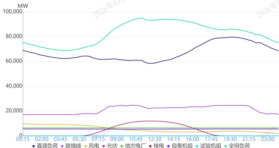
图 1 8月28日负荷及电源出力预测情况
