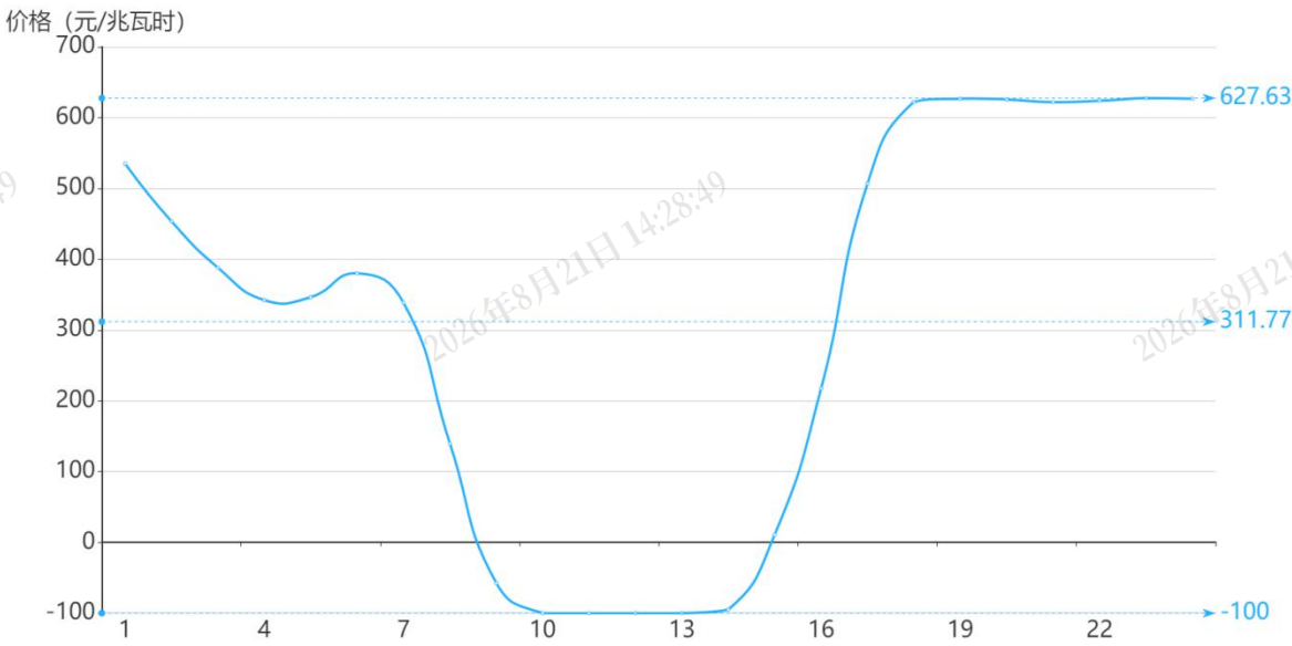
图 2 8 月 28 日日前市场用电侧价格
