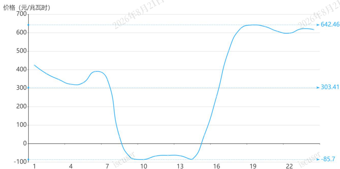
图3 8月28日实时市场用电侧价格
