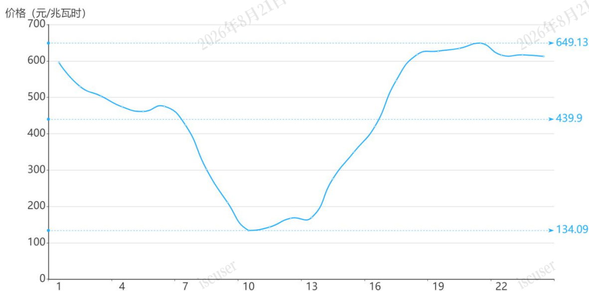
图3 8月30日实时市场用电侧价格
