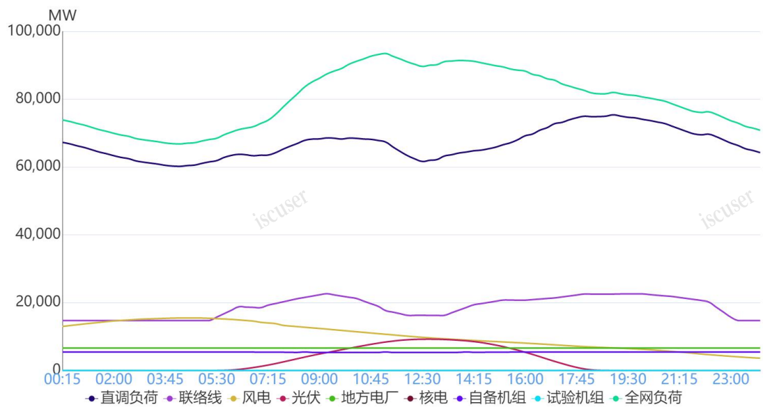
图 1 9 月 2 日负荷及电源出力预测情况
