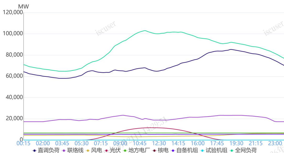
图 1 9月9日负荷及电源出力预测情况
