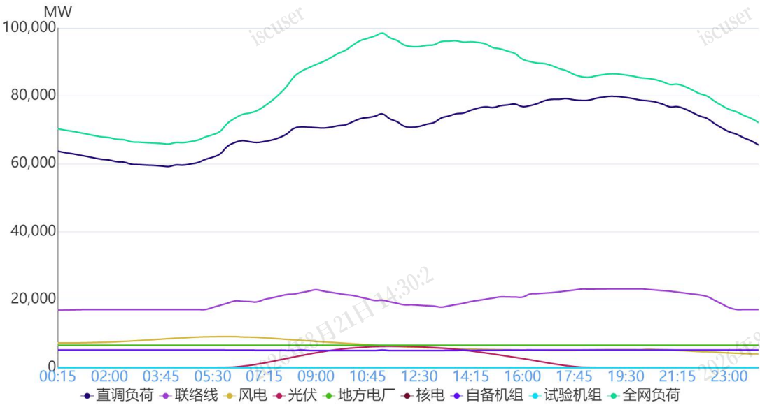
图1 9月12日负荷及电源出力预测情况
