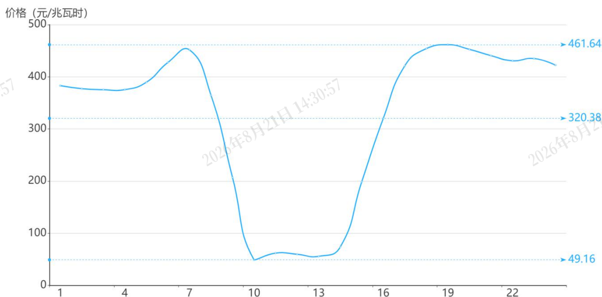
图 2 9 月 25 日日市场用电侧价格
