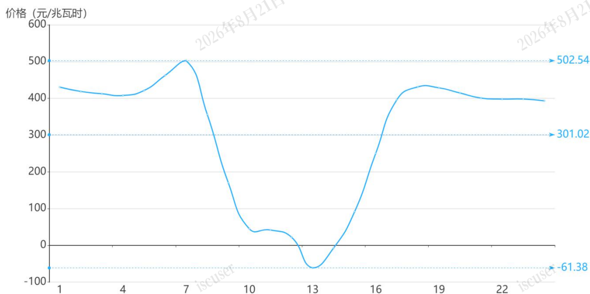
图3 9月24日实时市场用电侧价格
