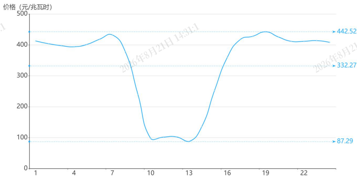
图 2 9 月 26 日日前市场用电侧价格
