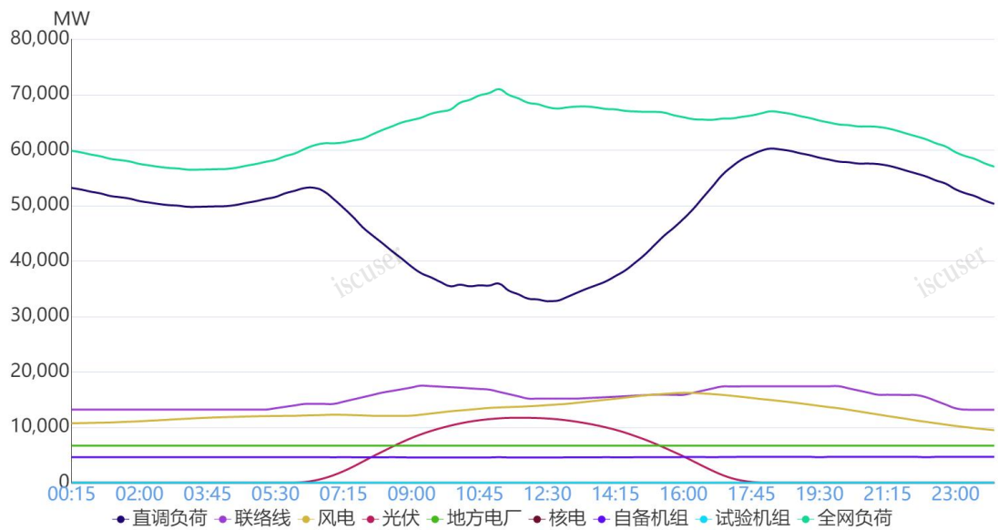
图 1 10 月 1 日负荷及电源出力预测情况
