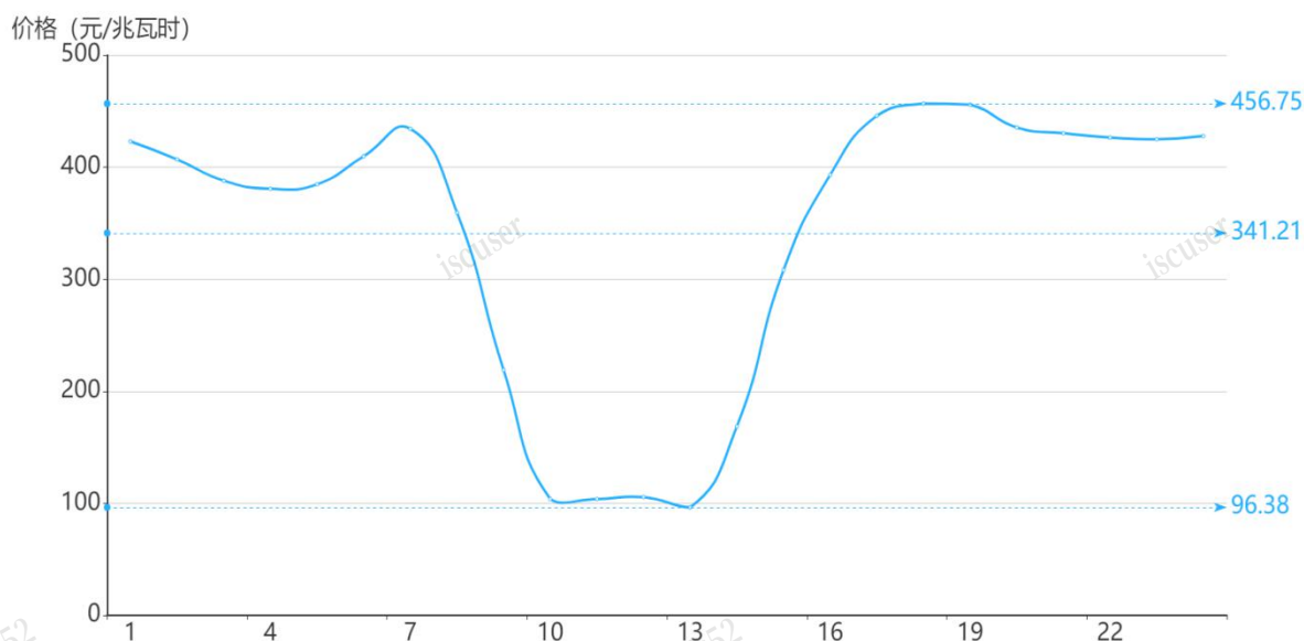
图2 10月9日日前市场用电侧价格
