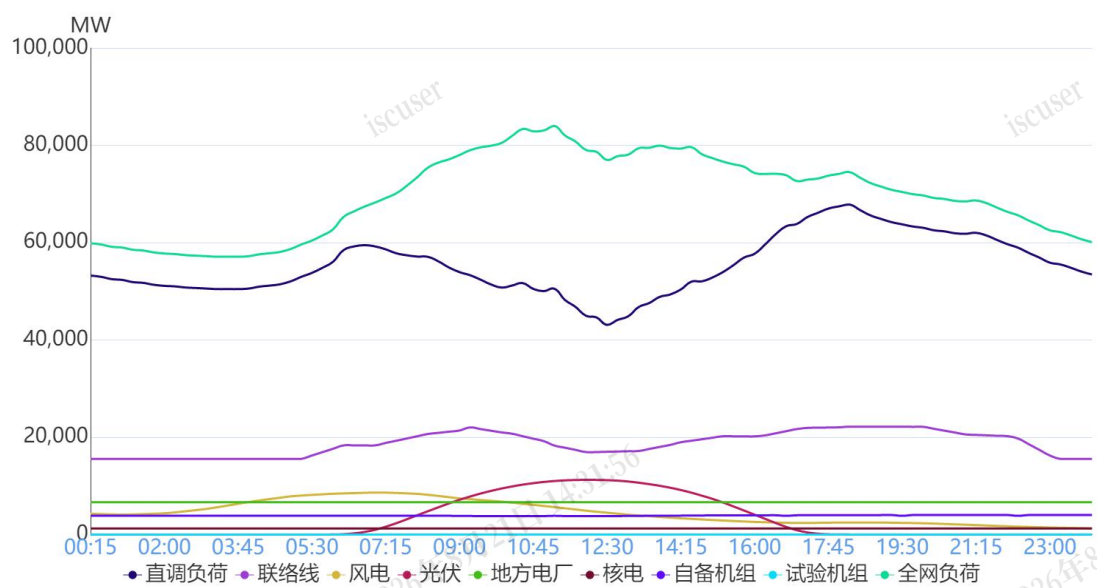
图 1 10月10日负荷及电源出力预测情况
