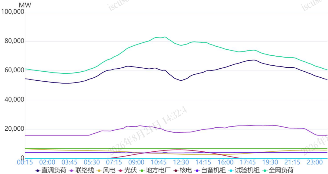
图 1 10月13日负荷及电源出力预测情况
