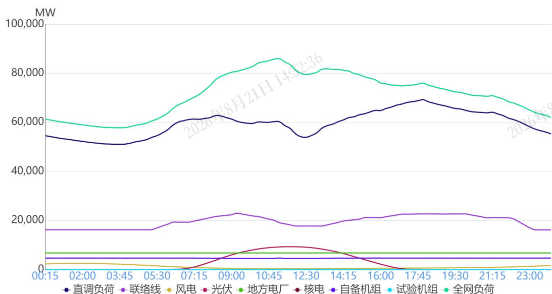
图 1 10月21日负荷及电源出力预测情况
