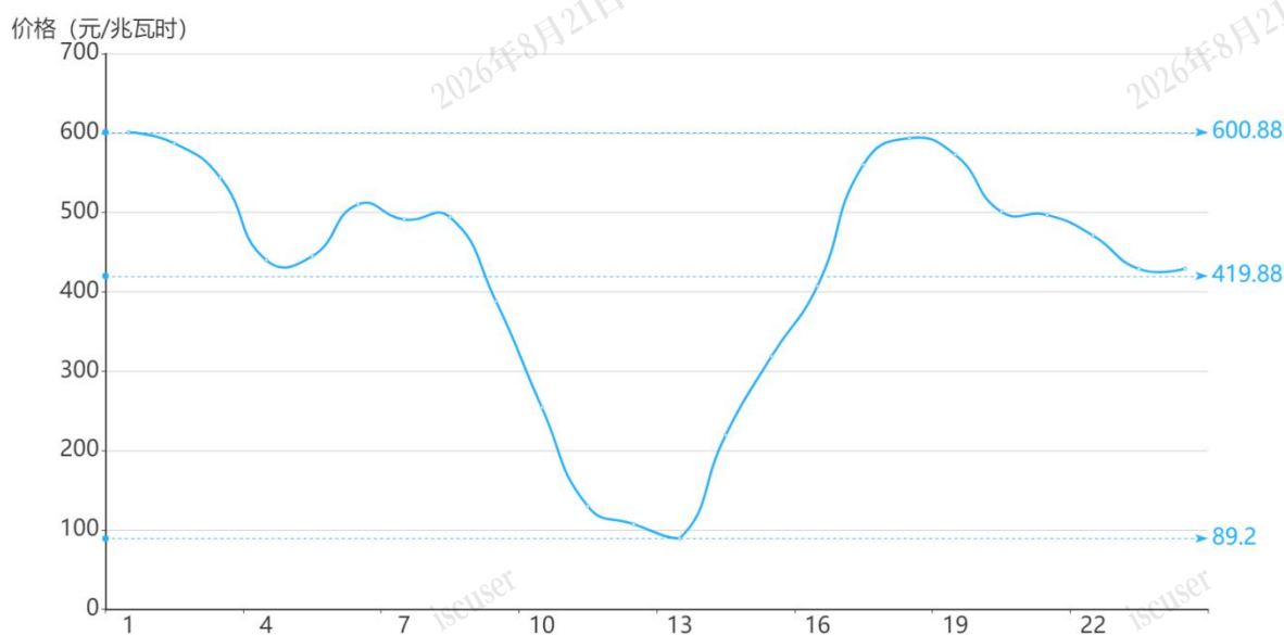
图3 10月27日实时市场用电侧价格
